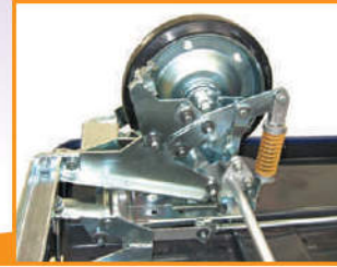
AS502HB-Sのアシスト部
