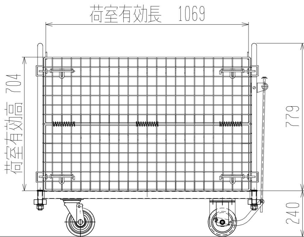
側面図(扉側)
